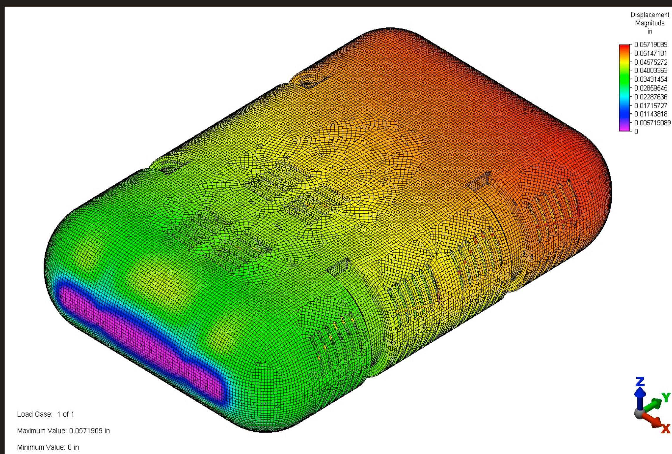
Bottom Impact Displacement
